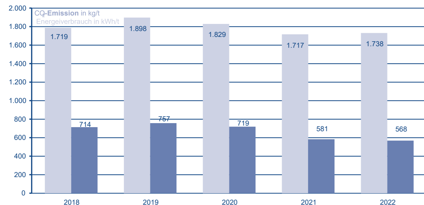
Diagramm 4: spezifischer Energieverbrauch in kWh/t netto und CO 2 -Emission in kg/t in der Kartonerzeugung
